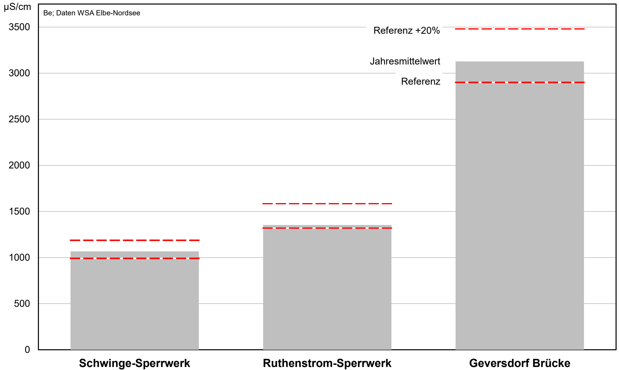
Jahresmittelwerte 2021 der Elektrischen Leitfähigkeit und die jeweiligen Referenzwerte
