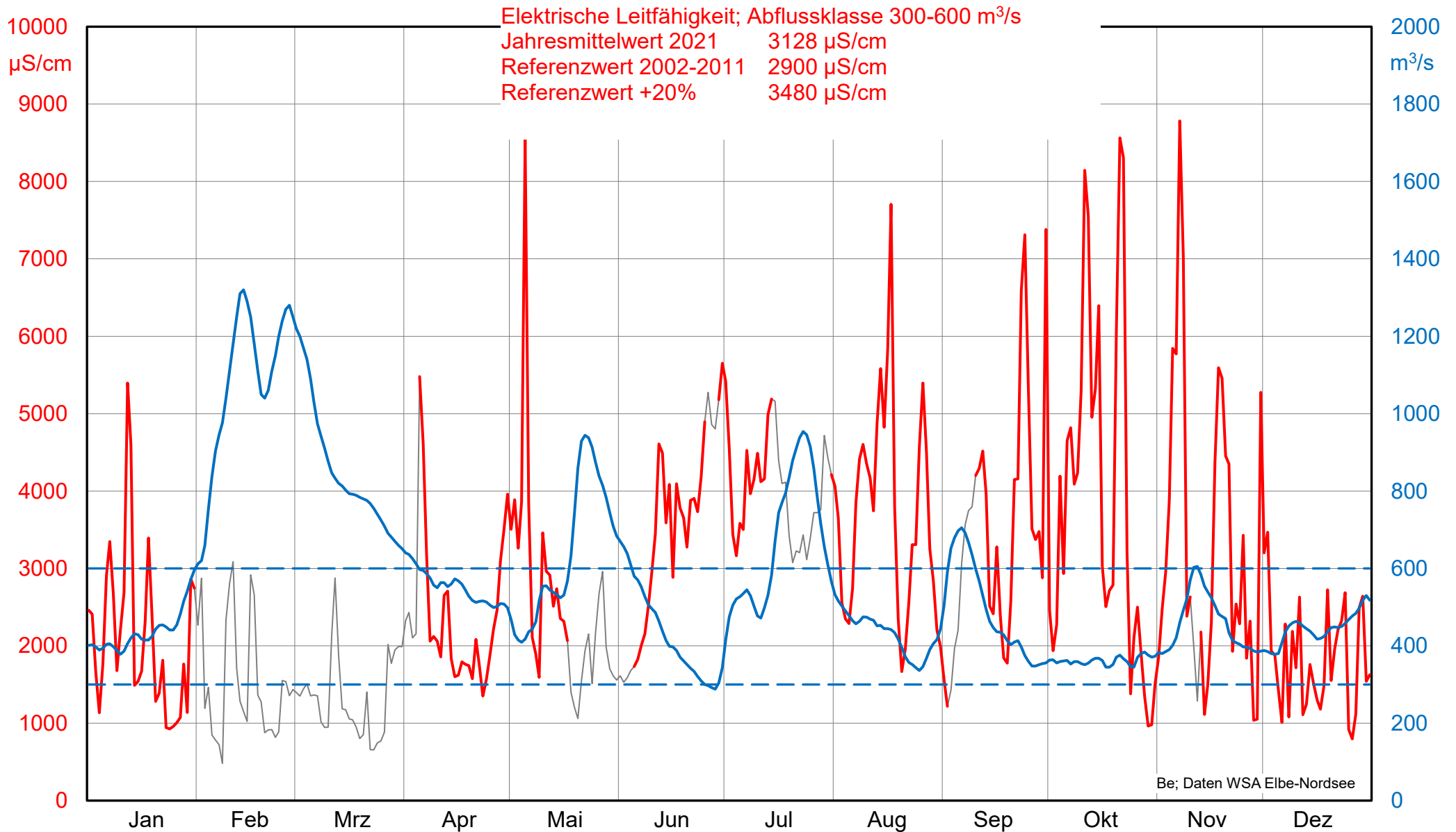
Elektrische Leitfähigkeit der Oste an der Brücke Geversdorf und der Abfluss der Elbe am Pegel Neu Darchau - 2021 Tagesmittelwerte
