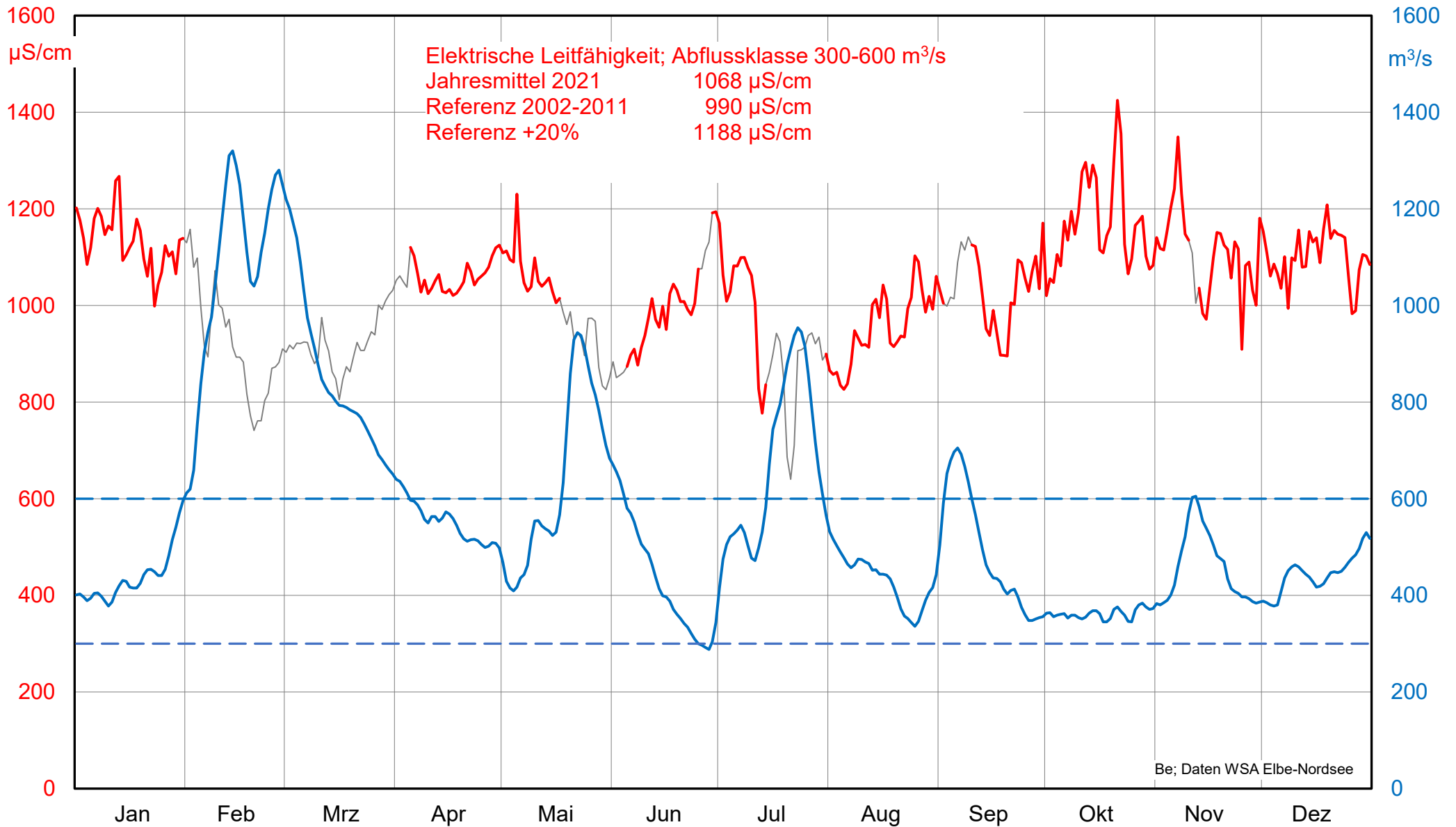
Elektrische Leitfähigkeit der Schwinge am Sperrwerk Stadersand und der Abfluss der Elbe am Pegel Neu Darchau - 2021 Tagesmittelwerte
