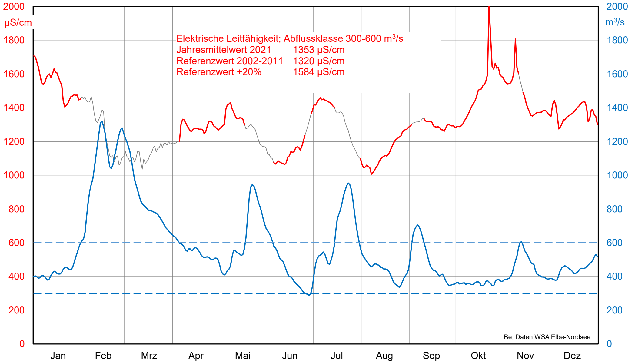
Elektrische Leitfähigkeit des Ruthenstroms am Sperrwerk Drochtersen und der Abfluss der Elbe am Pegel Neu Darchau - 2021 Tagesmittelwerte
