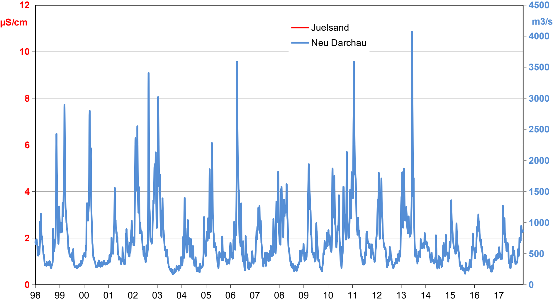
Tagesmittelwerte der el. Leitfähigkeit der Elbe bei Juelsand und der Abfluss am Pegel Neu Darchau - 1998-2017
