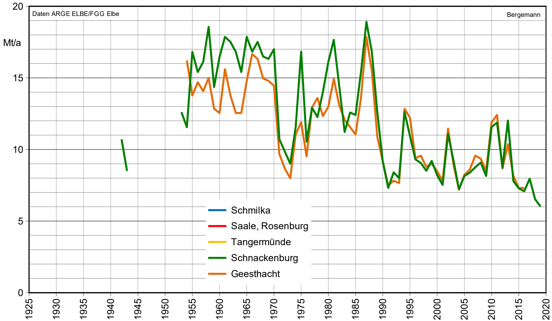
Salzfrachten [Mt/a] der Elbe – 1926 bis 2019
